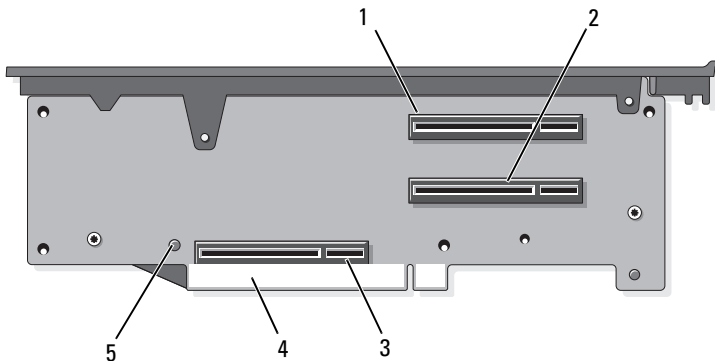
Figura 6-6. Componentes de la tarjeta vertical de expansión PCIe 1
