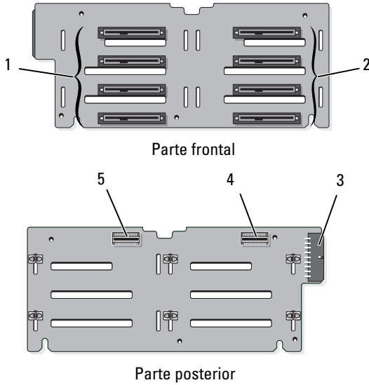
Figura 6-3. Placa de plano posterior SAS para unidades de disco duro de 2,5 pulgadas
