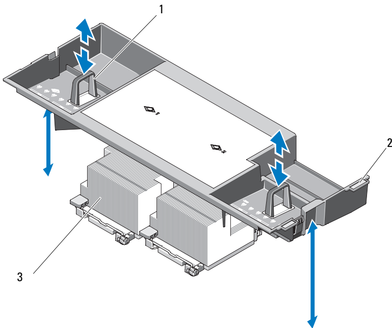
Figura 3-12. Extracción e instalación de la cubierta de refrigeración
