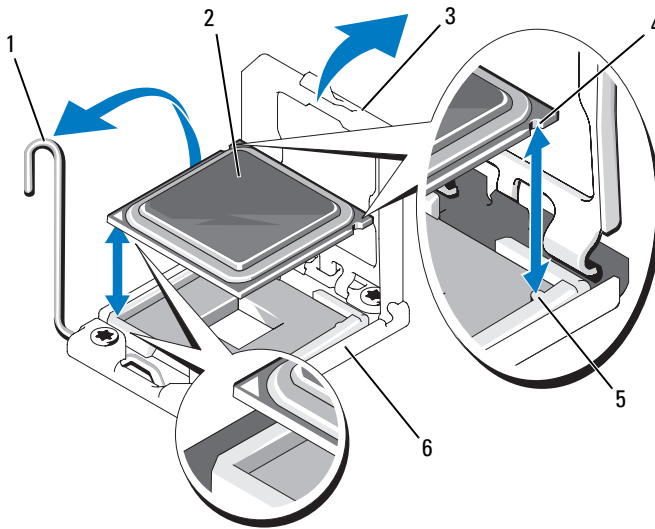
Figura 3-32. Instalación y extracción de un procesador
