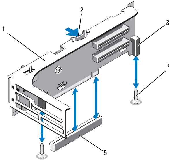
Figura 3-28. Extracción y colocación de la tarjeta vertical de expansión 2
