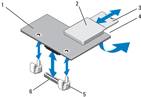
Figura 3-10. Extracción e instalación de la tarjeta iDRAC6 Enterprise
