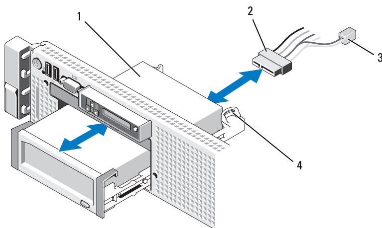
Figura 3-19. Extracción e instalación de la unidad de copia de seguridad en cinta
