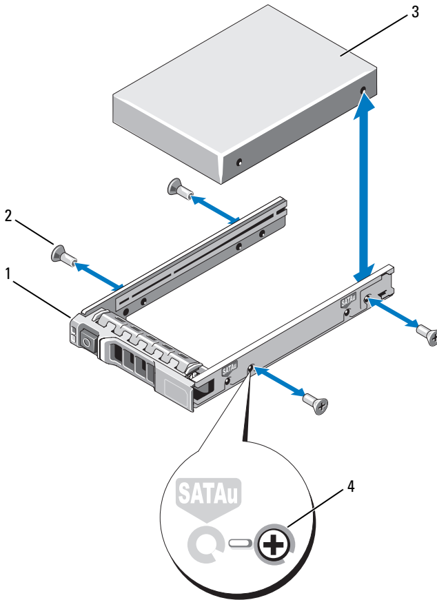
Figura 3-6. Instalación de una unidad de disco duro en un portaunidades
