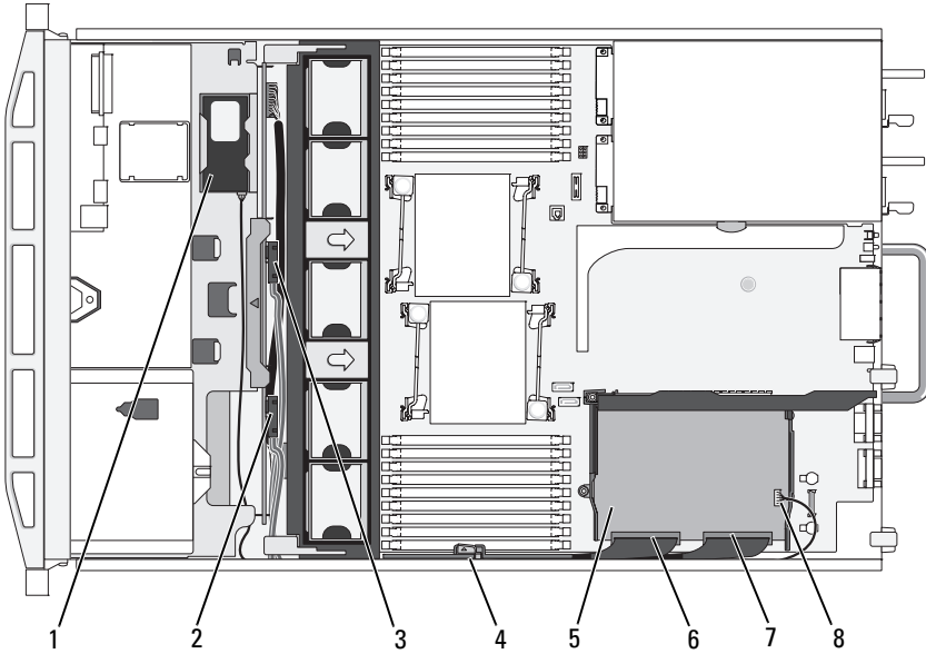
Figura 3-22. Cableado de la tarjeta controladora de almacenamiento (seis chasis de unidad de disco duro de 3,5 pulgadas)
