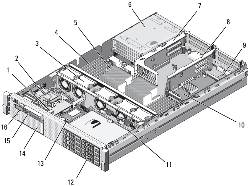
Figura 3-1. Interior del sistema (chasis de unidad de disco duro de 2,5 pulgadas)
