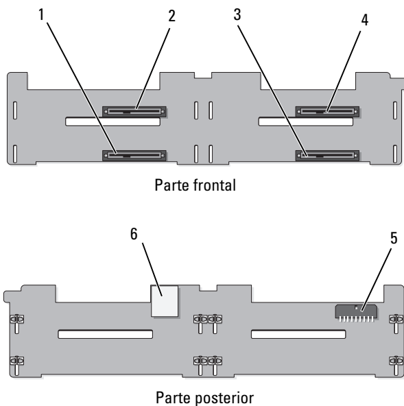
Figura 6-4. Placa de plano posterior SAS para unidades de disco duro de 3,5 pulgadas (4 ranuras)
