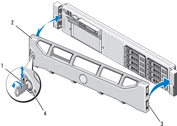
Figura 3-2. Extracción del embellecedor frontal
