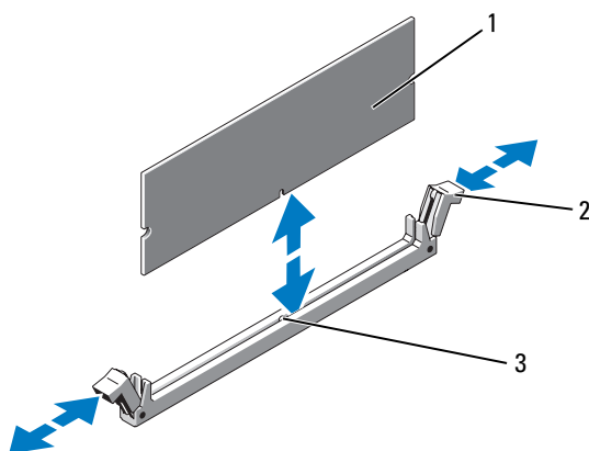
Figura 3-30. Instalación y extracción de un módulo de memoria
