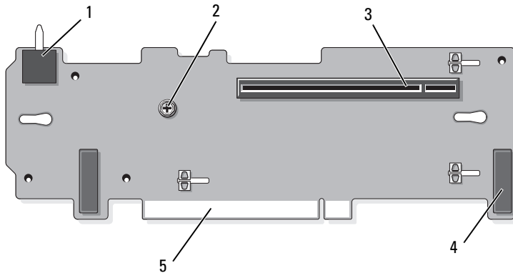
Figura 6-8. Componentes opcionales de la tarjeta vertical de expansión PCIe x16 2
