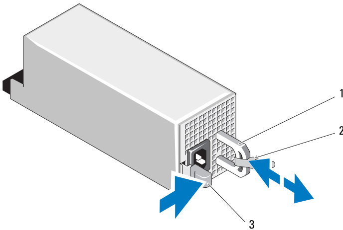
Figura 3-7. Extracción e instalación de una fuente de alimentación
