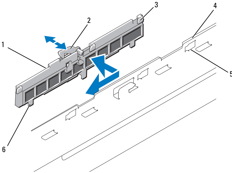
Figura 3-25. Extracción e instalación del soporte de retención de cables
