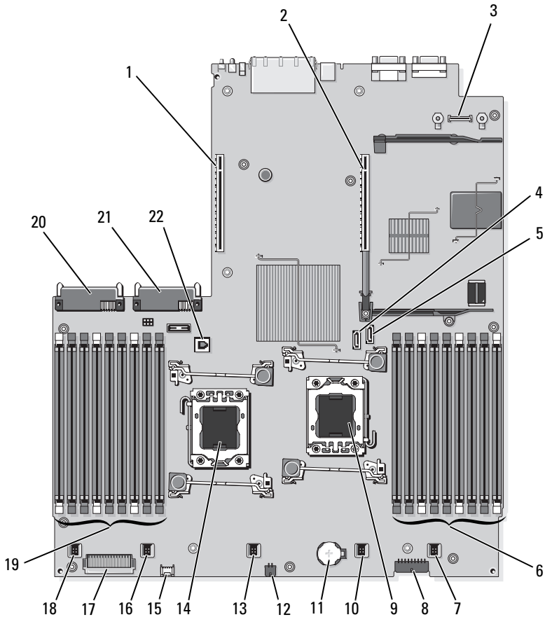
Figura 6-2. Conectores de la placa base
