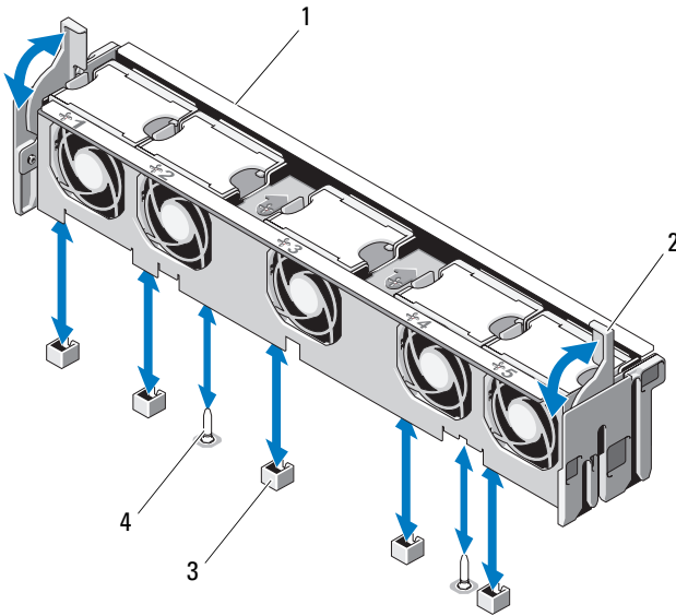
Figura 3-14. Extracción e instalación del soporte del ventilador del procesador
