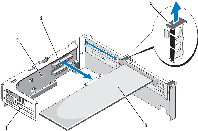
Figura 3-26. Extracción e instalación de una tarjeta de expansión
