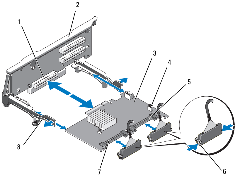
Figura 3-20. Instalación de una tarjeta controladora de almacenamiento
