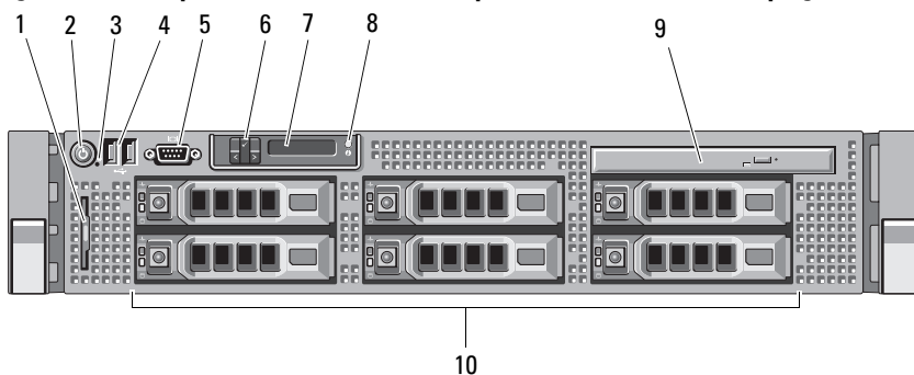
Figura 1-2. Componentes e indicadores del panel frontal (chasis de 3,5 pulgadas)
