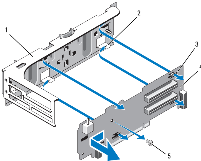
Figura 3-29. Extracción y colocación de la tarjeta vertical 2
