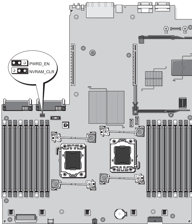
Figura 6-1. Puentes de la placa base
