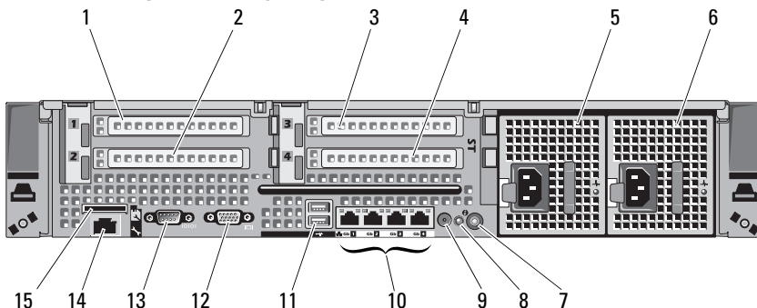
Figura 1-5. Componentes del panel posterior
