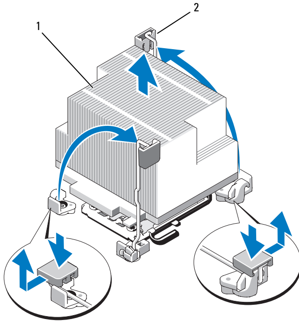
Figura 3-31. Instalación y extracción del disipador de calor
