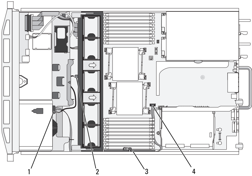
Figura 3-17. Enrutamiento del cable de la unidad óptica (chasis de unidad de disco duro de 3,5 pulgadas)
