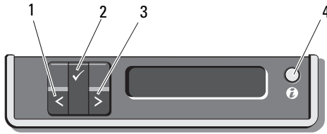
Figura 1-3. Componentes del panel LCD
