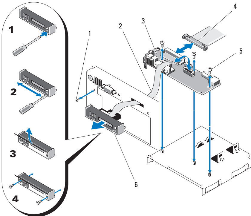
Figura 3-34. Extracción e instalación del panel de control
