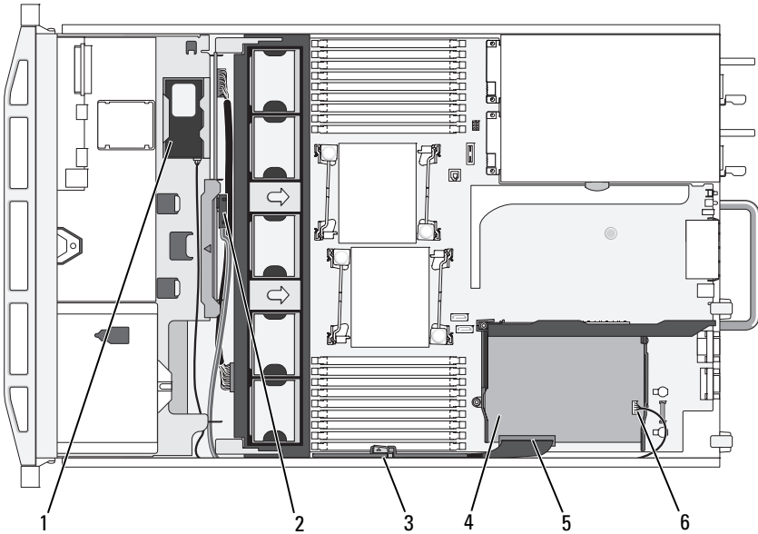
Figura 3-23. Cableado de la tarjeta controladora de almacenamiento (cuatro chasis de unidad de disco duro de 3,5 pulgadas)
