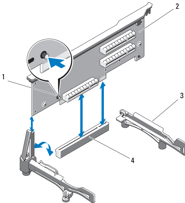
Figura 3-27. Extracción y colocación de la tarjeta vertical de expansión 1
