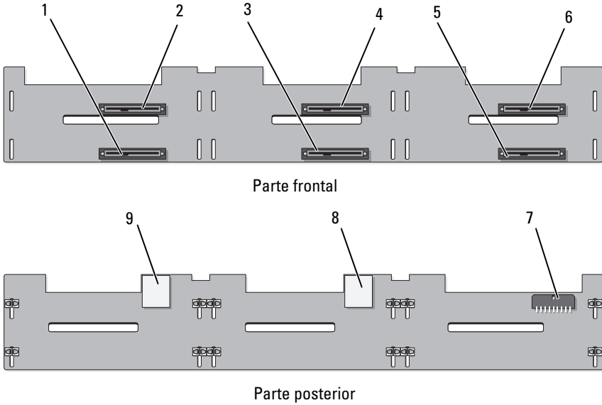
Figura 6-5. Placa de plano posterior SAS para unidades de disco duro de 3,5 pulgadas (6 ranuras)
