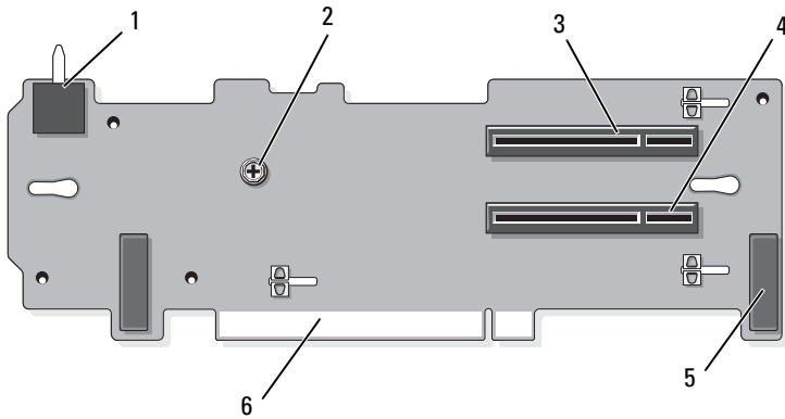
Figura 6-7. Componentes de la tarjeta vertical de expansión PCIe 2 estándar
