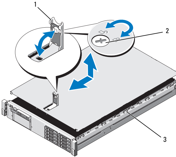
Figura 3-3. Extracción e instalación de la cubierta
