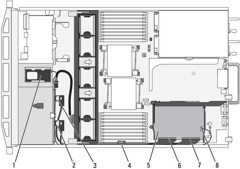
Figura 3-21. Cableado de la tarjeta controladora de almacenamiento (chasis de unidad de disco duro de 2,5 pulgadas)
