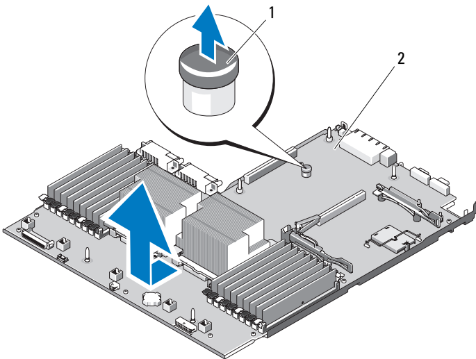
Figura 3-36. Extracción de la placa base
