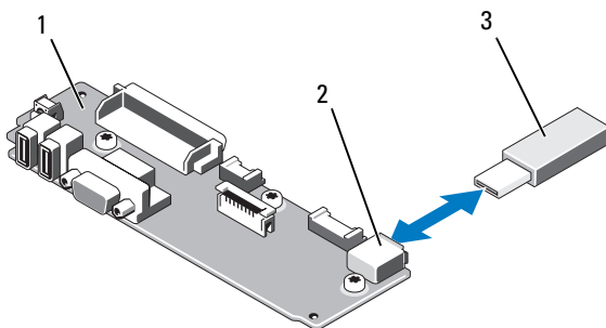
Figura 3-9. Extracción o instalación de una memoria USB
