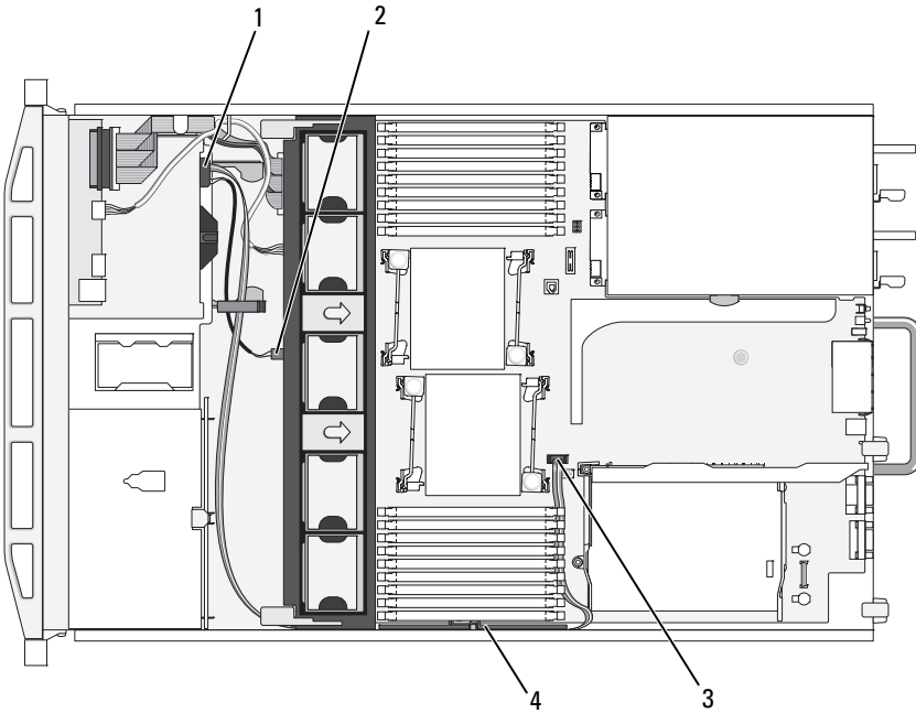
Figura 3-16. Enrutamiento del cable de la unidad óptica (chasis de unidad de disco duro de 2,5 pulgadas)
