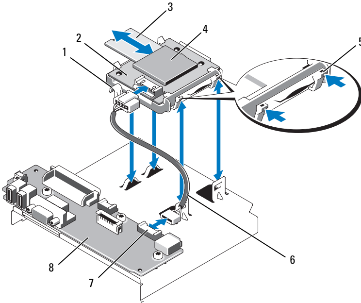
Figura 3-8. Extracción e instalación del módulo SD interno
