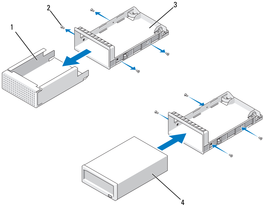
Figura 3-18. Preparación de la unidad de copia de seguridad en cinta y de la bandeja (sólo chasis de unidad de disco duro de 3,5 pulgadas)
