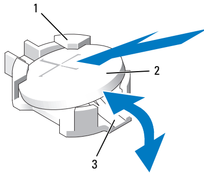
Figura 3-33. Sustitución de la batería del sistema
